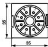
JQX-10F-2Z
